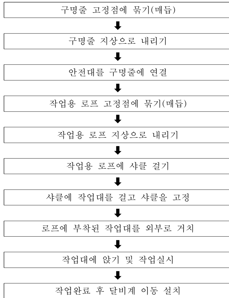
<그림 3> 작업의자형 달비게 작업순서
